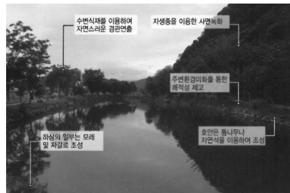
자연생태경관계획 예시(생태연못 및 습지)
