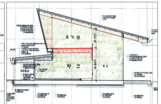
단면 대안
