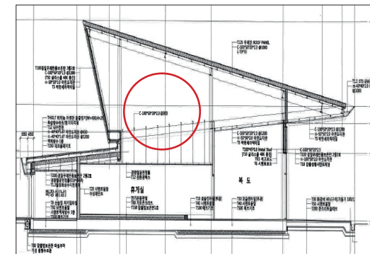
기본 단면 계획안
