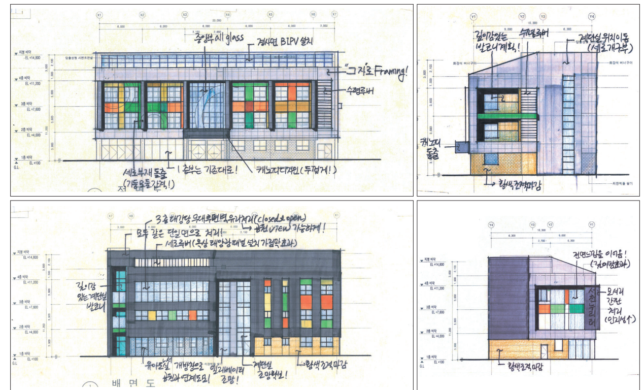
제시안
