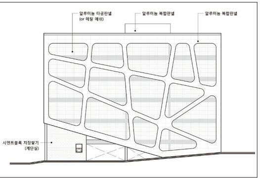
컨설팅 후(남측면도)
