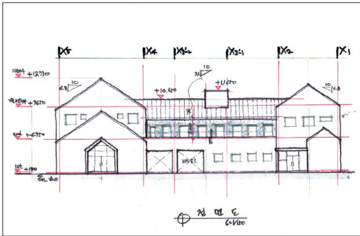
수정 제안안(정면도)
