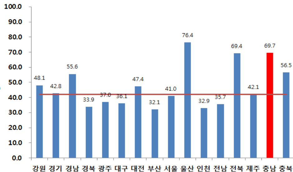
다중이용시설의 겨울철 라돈 농도 현황(2010년)
