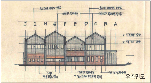
입면계획 대안 2(정면도/우측면도)
