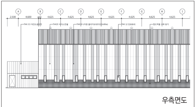
입면계획 대안 1(정면도/우측면도)
