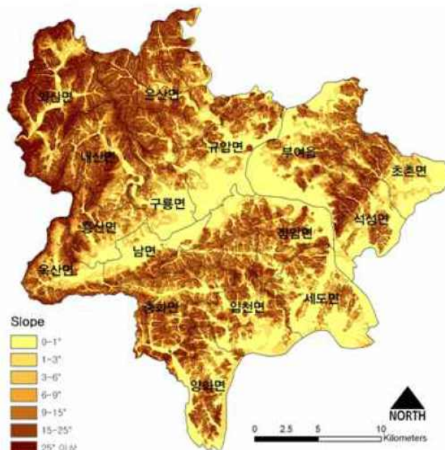
〈그림 3〉 부여군 경사도
