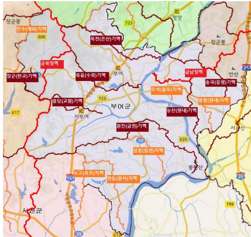
<그림 1> 부여군 산맥 분포
