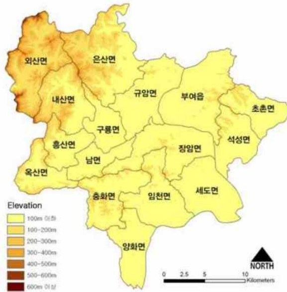
〈그림 2〉 부여군 표고도
