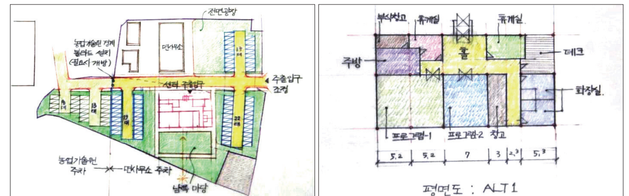
배치/평면계획 대안 1
