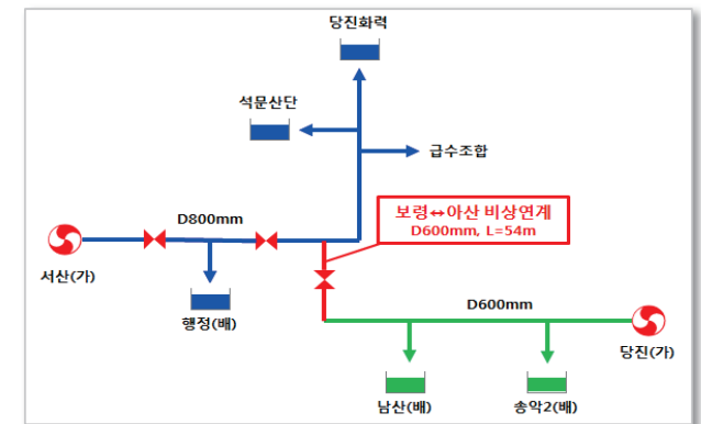
[ 당진계통 비상연계시설 ]
