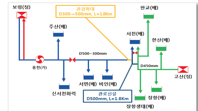
[ 서천·보령계통 비상연계시설 ]
