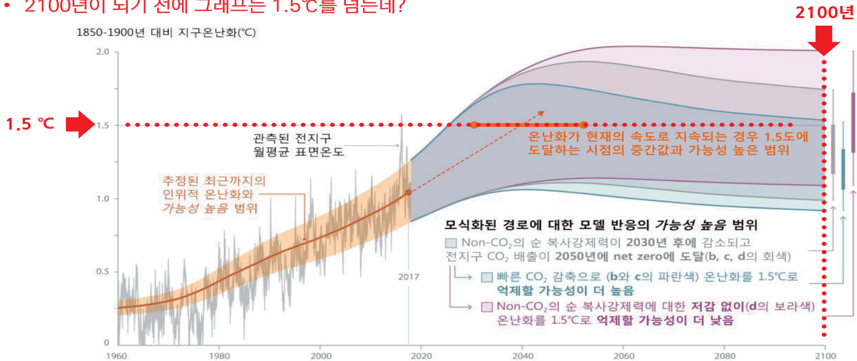
<그림> 관측된 전지구 기온변화와 모식화된 인간활동에 의한 배출 및 강제력 경로에 따른 모델 반응(IPCC SR15, 2018)
